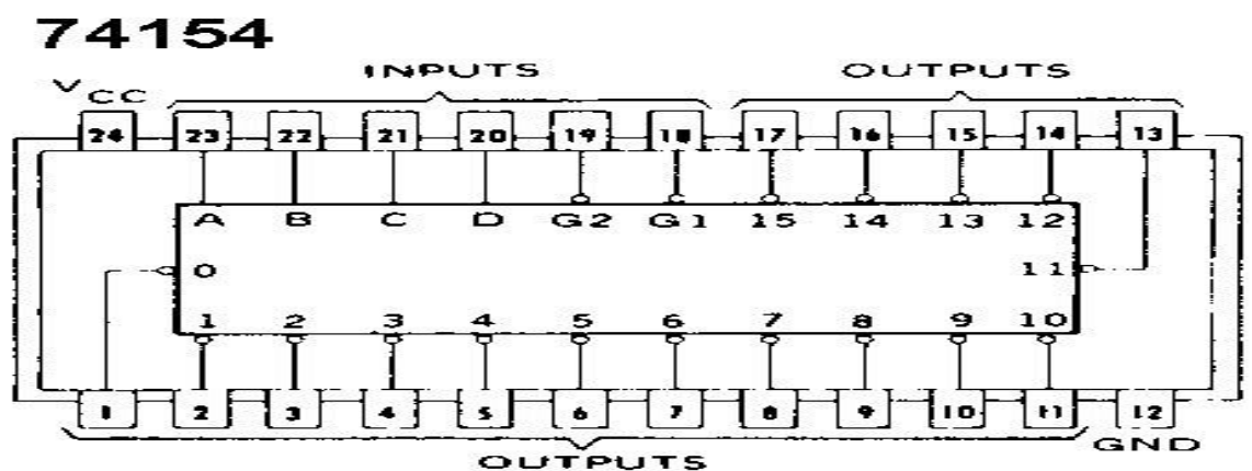
Fig. 8: 74154
